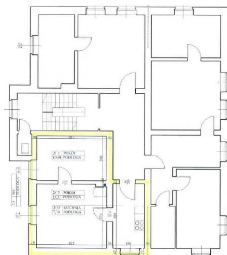
Rzut piętra
